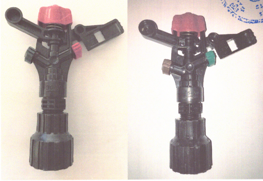
AKONA Çift Memeli Döner Yağmurlama Başlıkları
