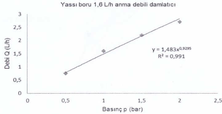
Şekil 2. Damlatıcı basınç – debi değişimi
