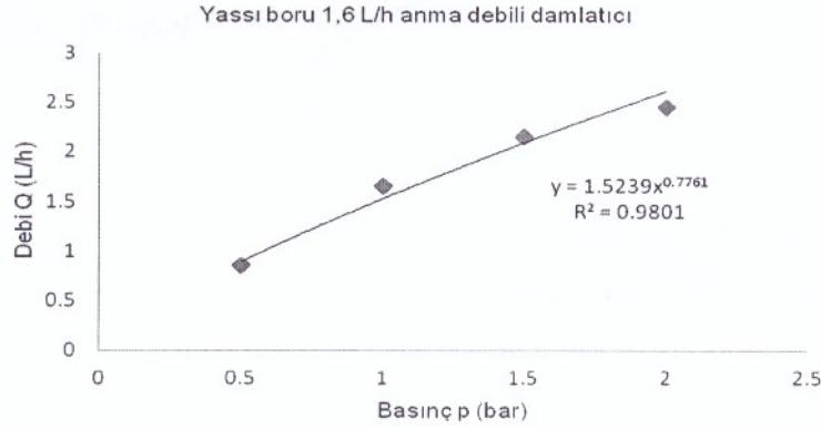
Şekil 2. Damlatıcı basınç – debi değişimi
