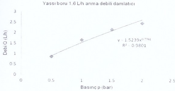
Şekil 1. Damlatıcı basınç – debi değişimi
